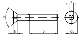
mit Innensechskant
