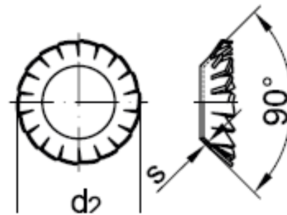
Form V = versenkt
