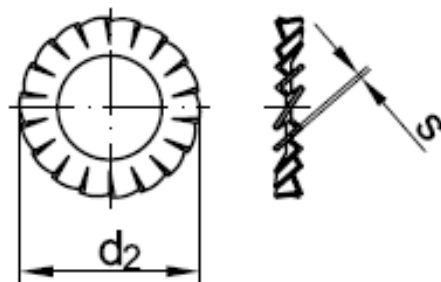
Form A = außengezahnt
